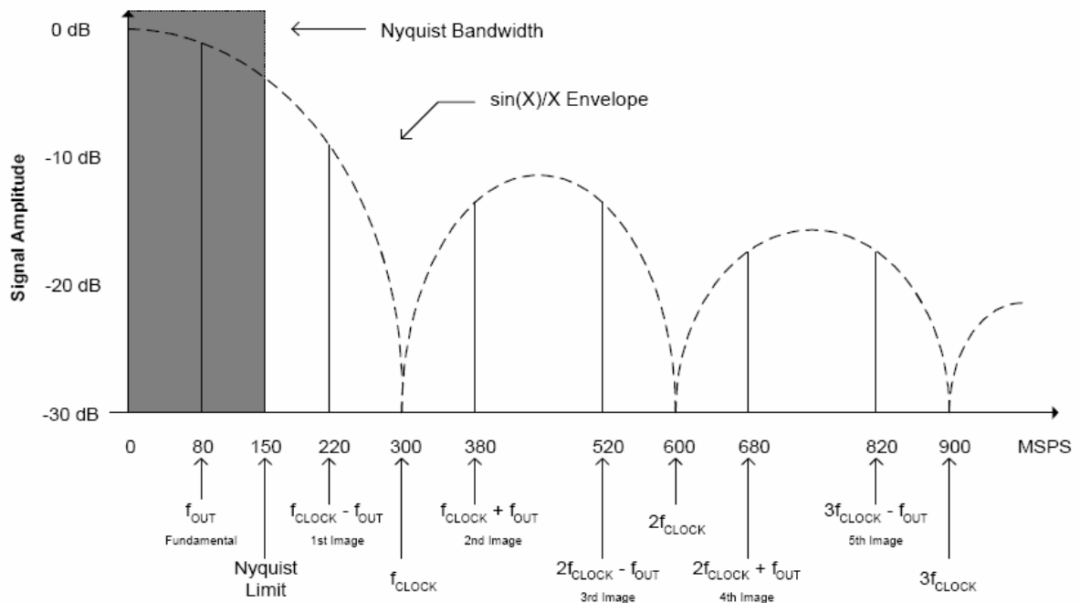
图 1. 300M 主频, 80M 输出 DDS 频谱
