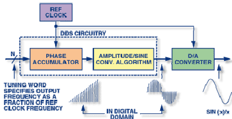
图 1, DDS 的结构
