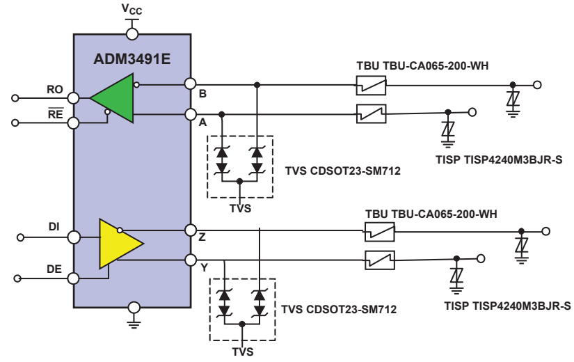
Protection Scheme 2—TVS/TBU/TISP
