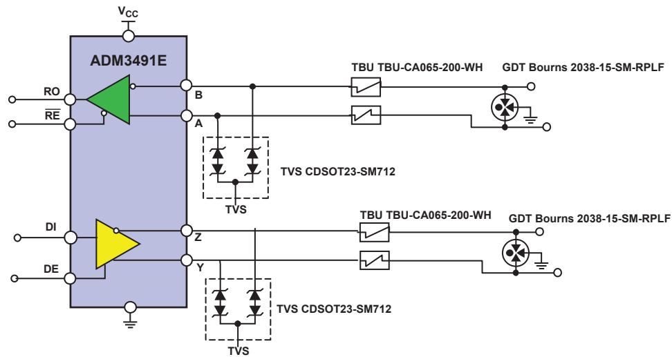
Protection Scheme 3—TVS/TBU/GDT
